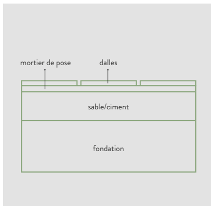
Coupe pour un placement traditionnelle
