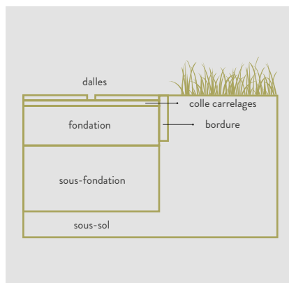
Coupe pour une allée
