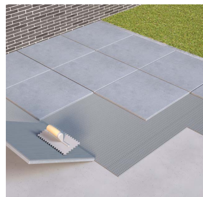
Placement dalles par encollage double avec colle pour carrelages
